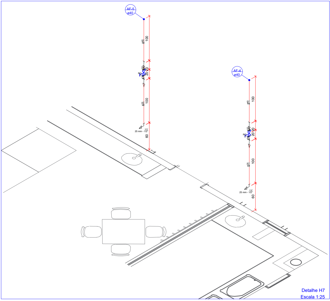
Detalhe H7 Escala 1:25
