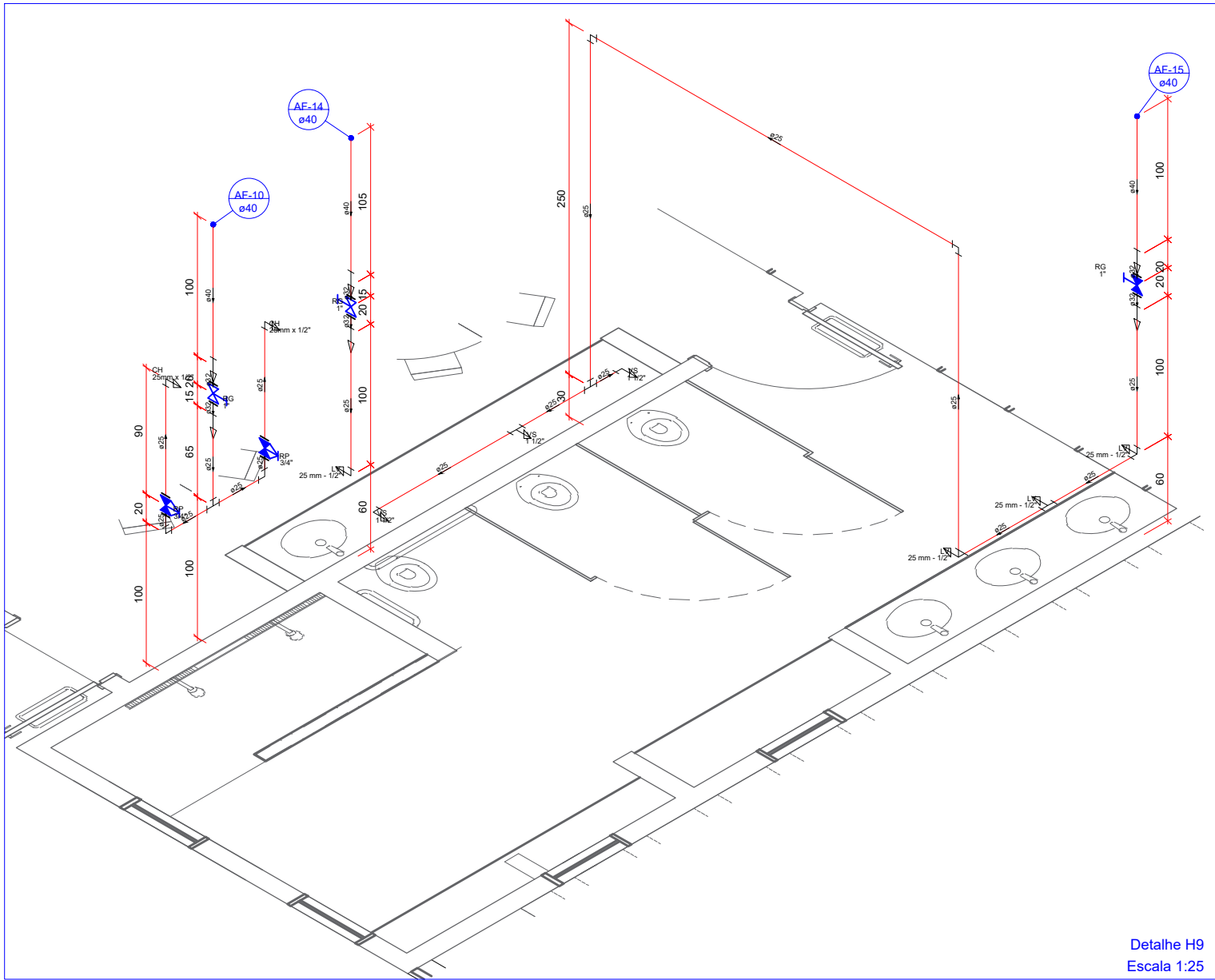
Detalhe H9 Escala 1:25
