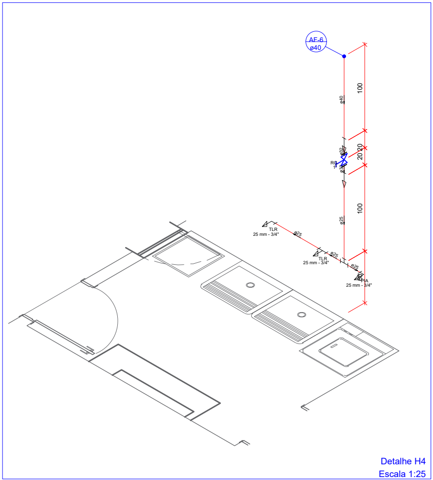
Detalhe H4 Escala 1:25
