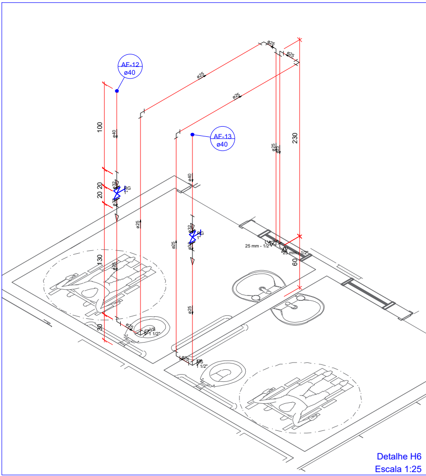
Detalhe H6 Escala 1:25
